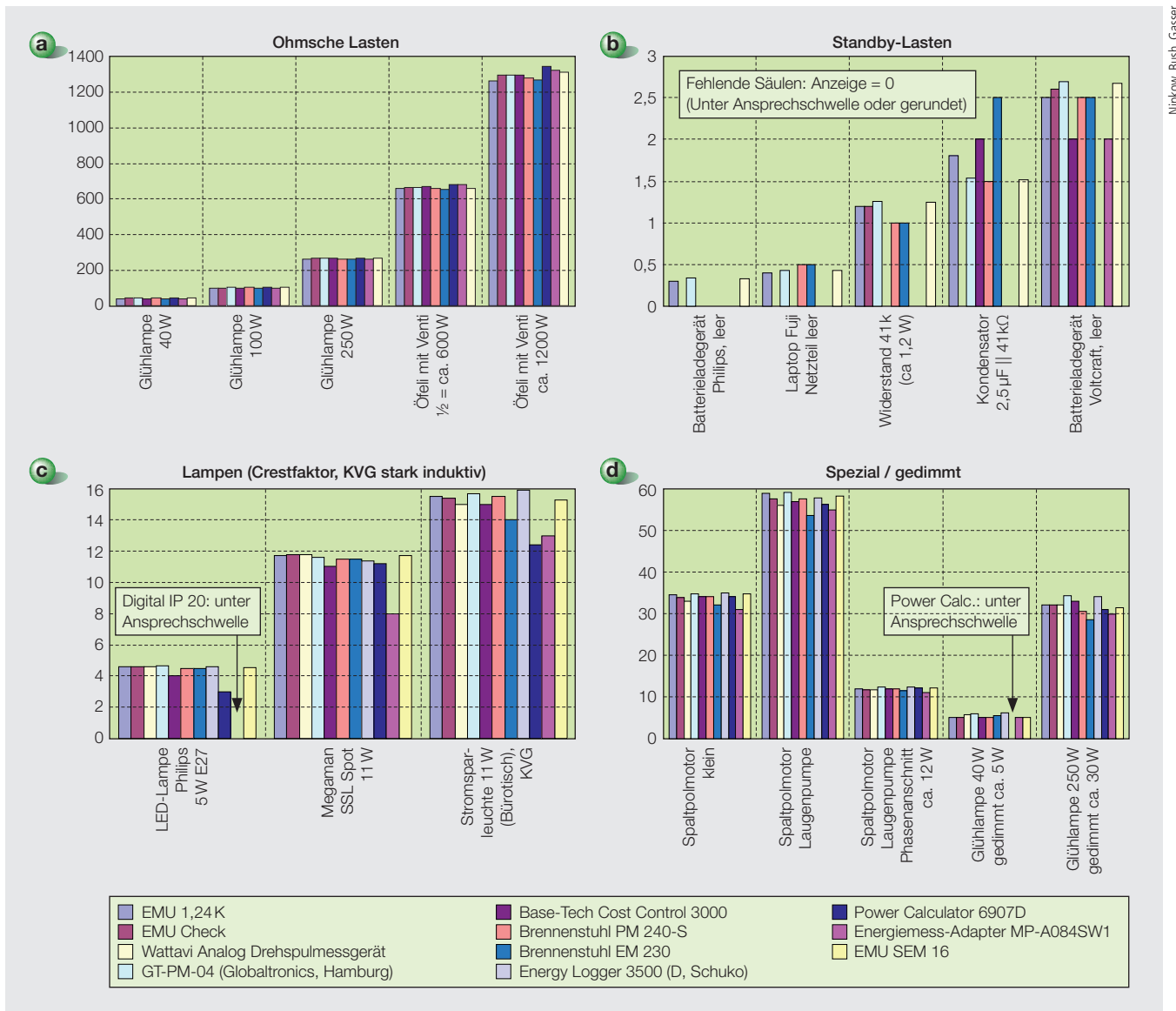
Bild 1 Auswertung der Leistungsanzeigen nach Lasten-Kategorien.
