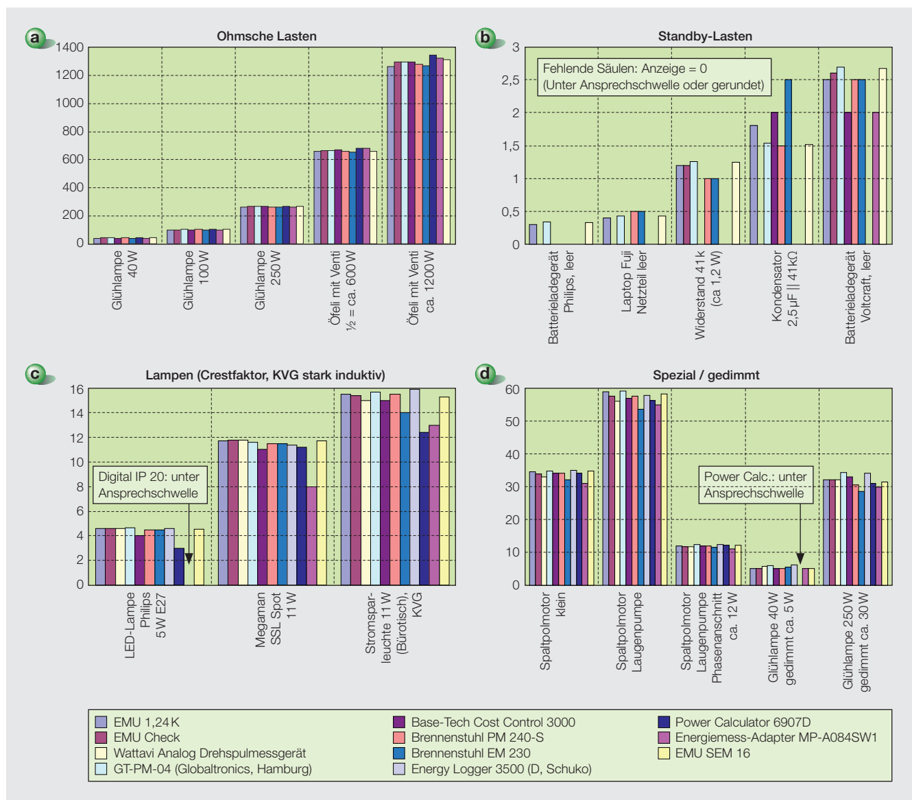
Bild 1 Auswertung der Leistungsanzeigen nach Lasten-Kategorien.
